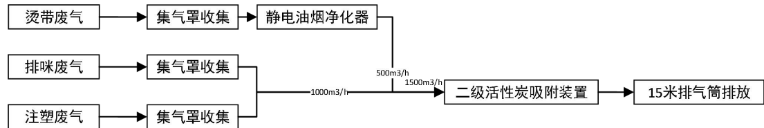
图 4-1 废气处理工艺
