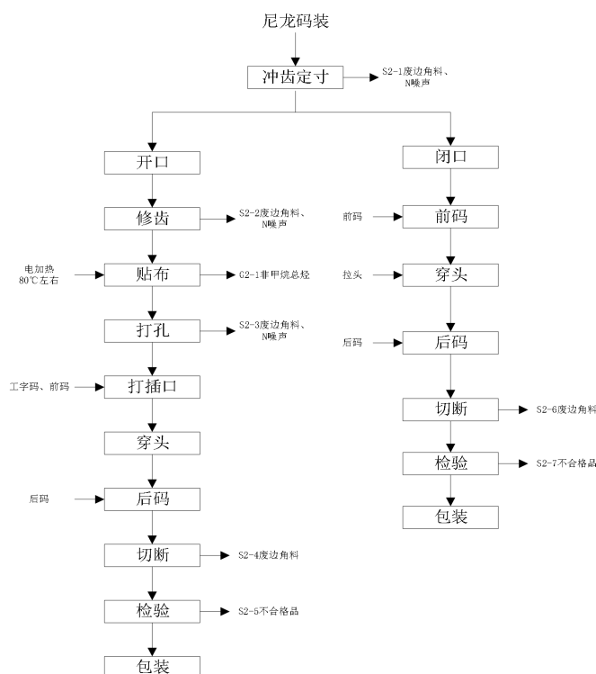
图 2-2 尼龙拉链生产工艺流程图
