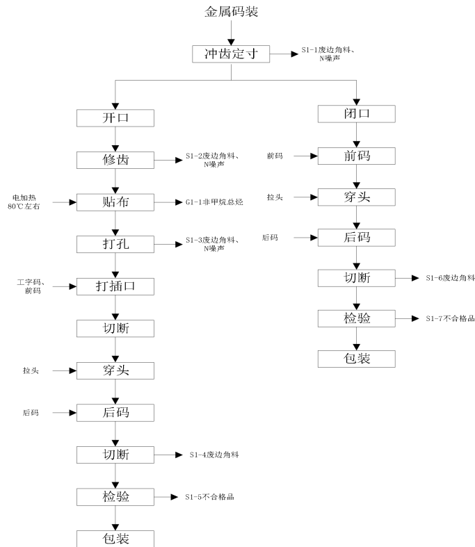
图 2-1 金属拉链生产工艺流程图
