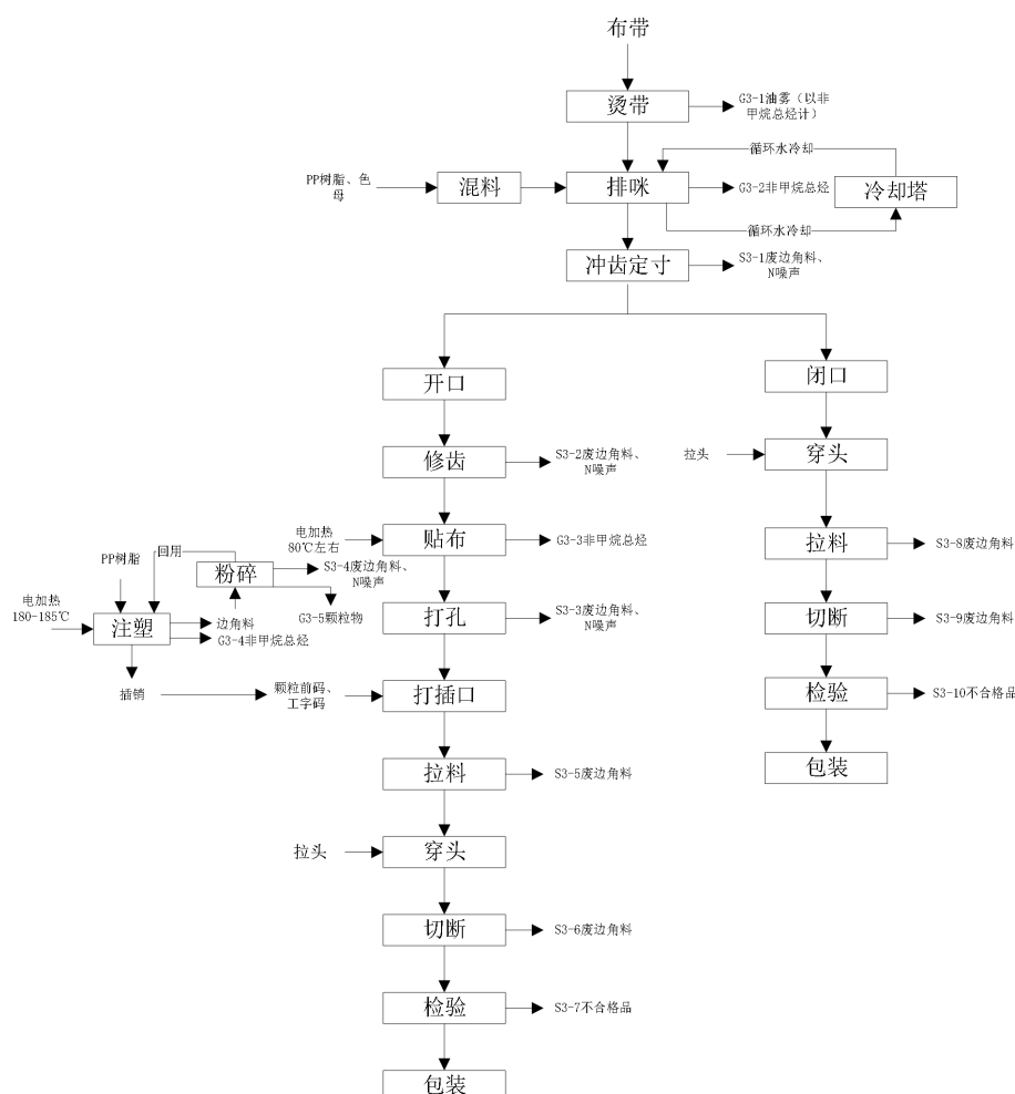
图 2-3 树脂拉链生产工艺流程图
