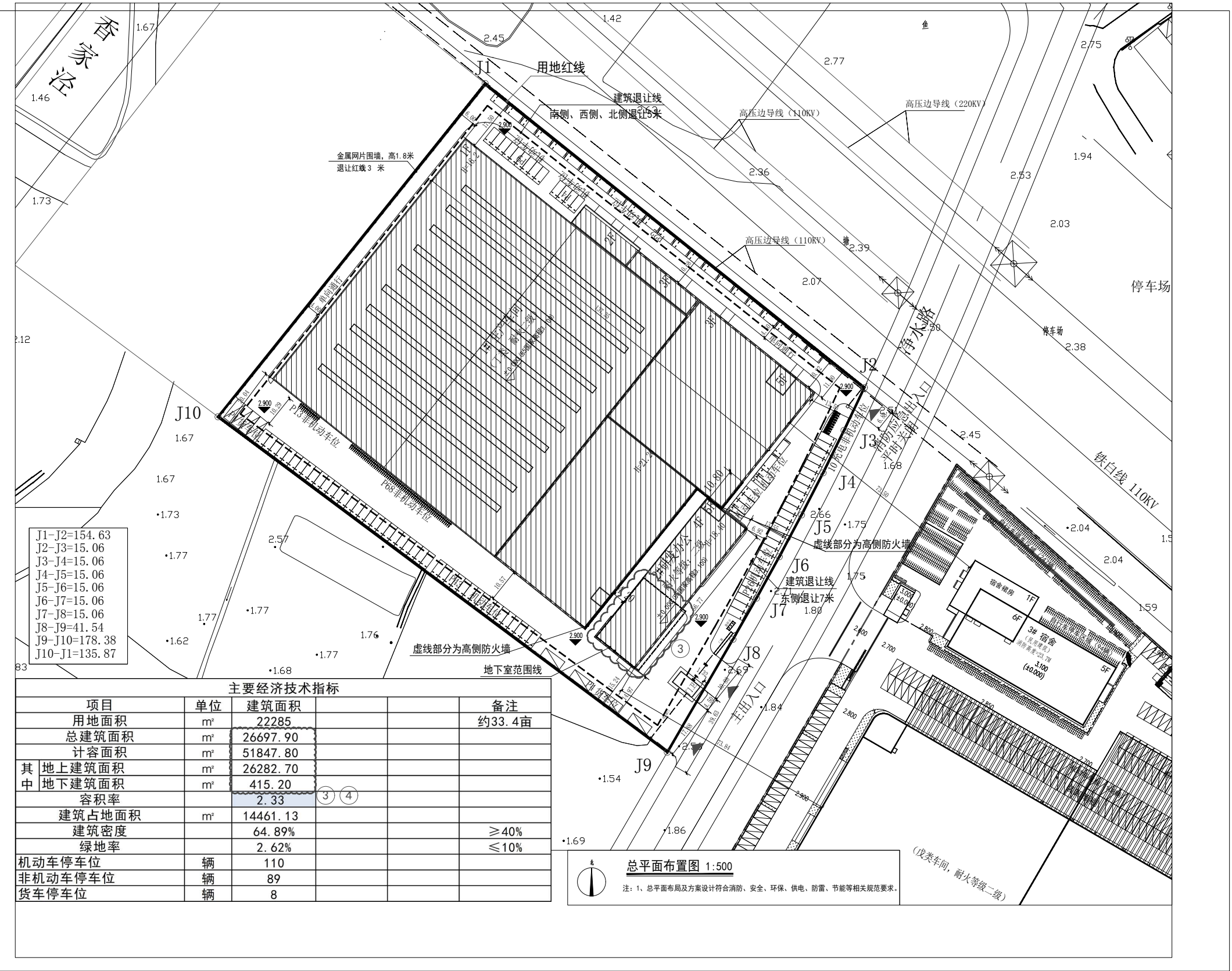
1#生产车间
